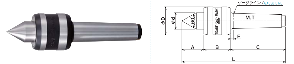
寸法表 / DIMENSIONS TABLE 単位 / UNIT mm
