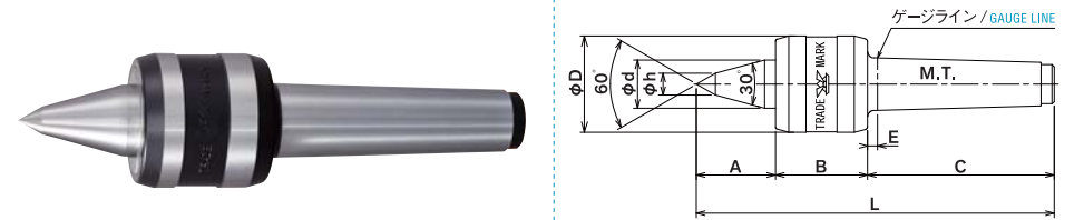
寸法表 / DIMENSIONS TABLE 単位 / UNIT mm
